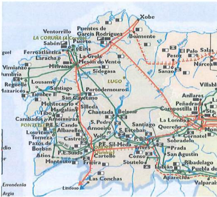
Esquema xeral da Rede Eléctrica Nacional na Comunidade Autónoma Galega.
